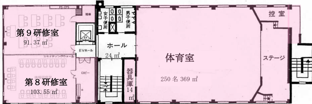
3 階平面図
